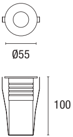
EST704
