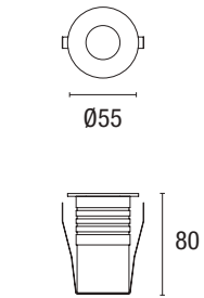
EST700 / EST 701
